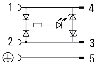
Схема соединений
