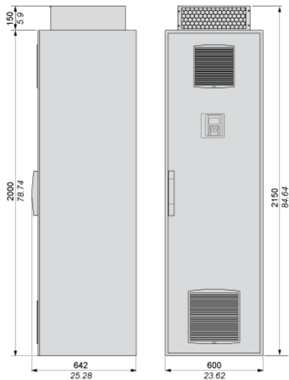
Rechtsseitige Ansicht und Vorderansicht
