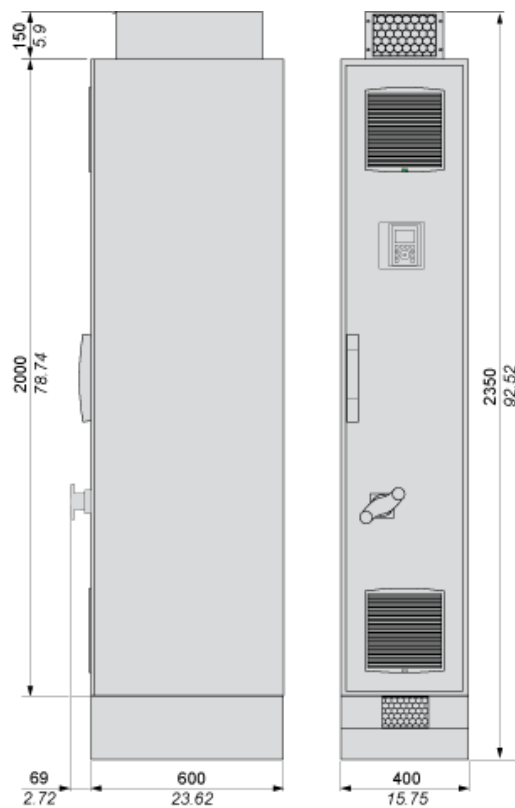
Rechtsseitige Ansicht und Vorderansicht
