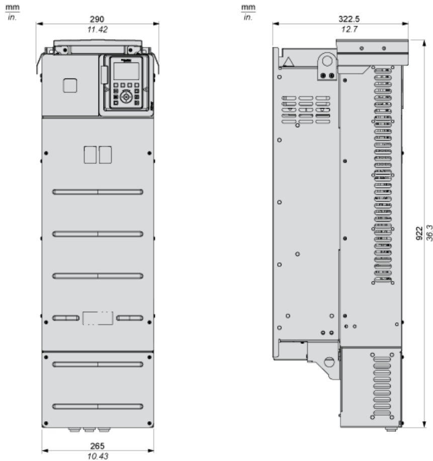
Vorderansicht und linksseitige Ansicht
