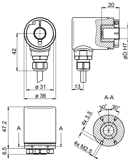
EAM360R, Kabel ohne Statorkupplung
