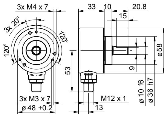
EAM580-SC mit Flanschdose M12
