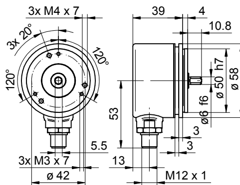
EAM580-SY mit Flanschdose M12
