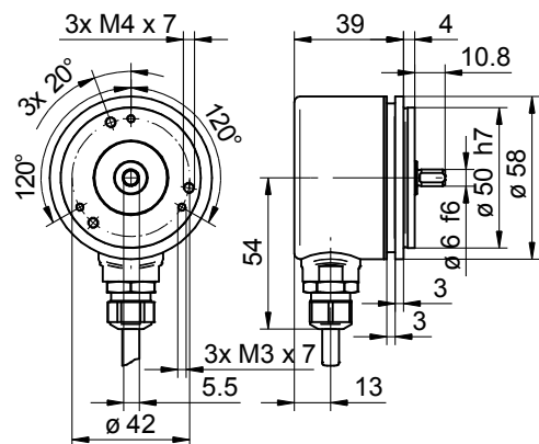
EAM580-SY mit Kabel
