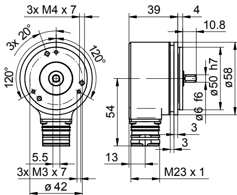
EAM580-SY mit Flanschdose M23
