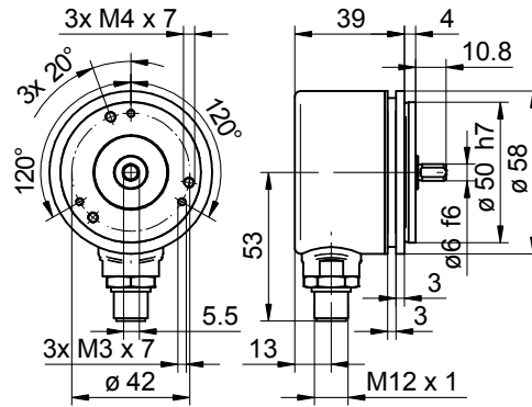
EAM580-SY mit Flanschdose M12
