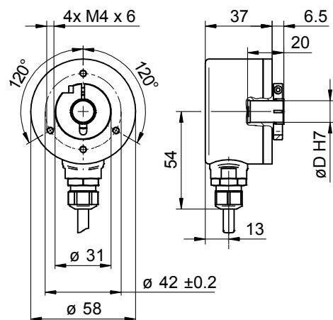
EAM580R, Kabel ohne Statorkupplung
