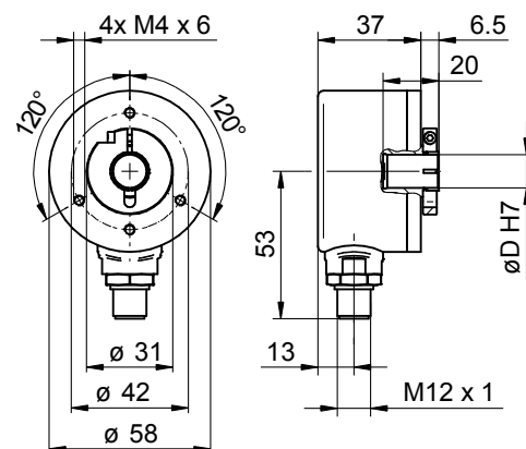
EAM580R, M12 ohne Statorkupplung
