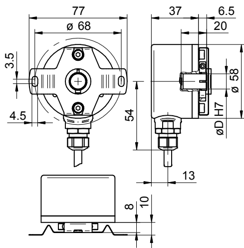
EAM580R, Kabel mit Statorkupplung
