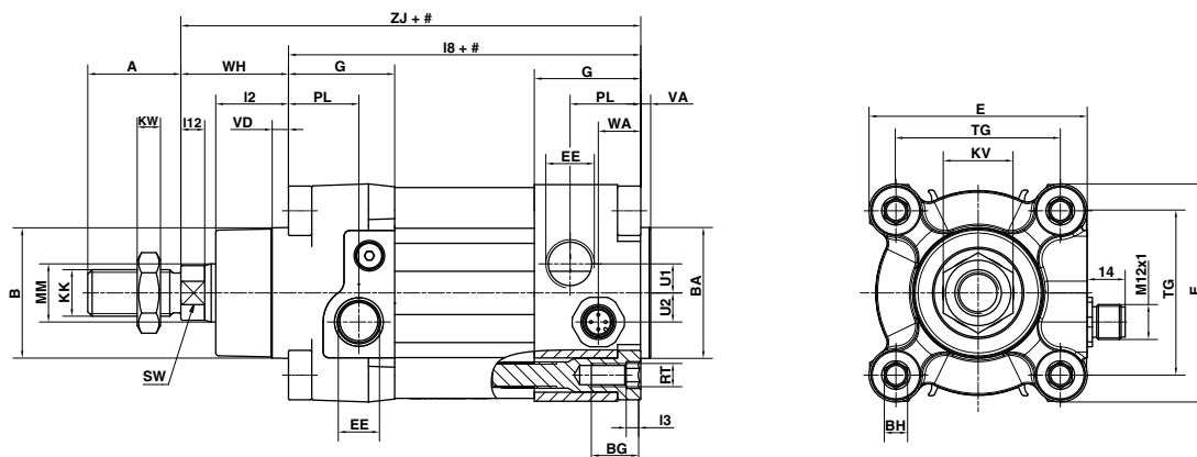
PSA/802040/F1 - PSA/802063/F1 ( \varnothing 40 ... 63 mm)
