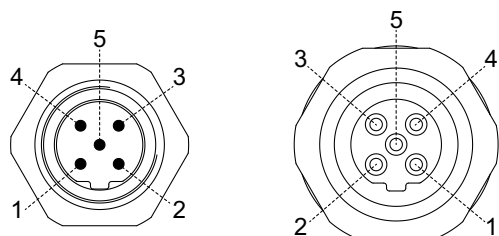
Stecker M12 (Stift, A 2) ) 5-polig, B-codiert
