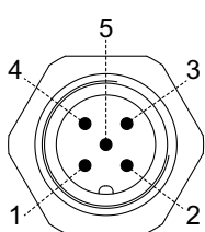
Stecker M12 (Stift, A 1) ) 5-polig, A-codiert
