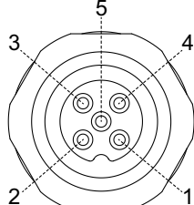
Stecker M12 (Buchse, A 2) ) 5-polig, A-codiert
