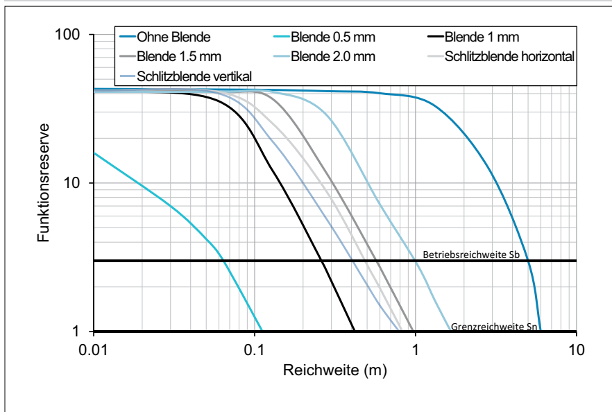
Funktionsreservekurve
