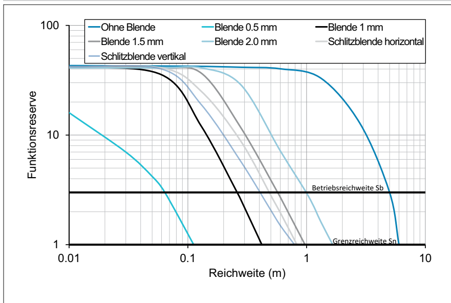
Funktionsreservekurve
