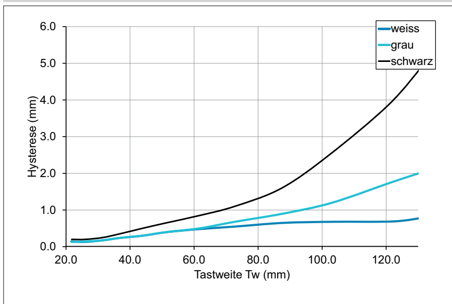
Hysteresekurve
