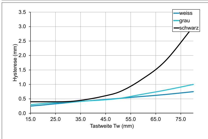
Hysteresekurve
