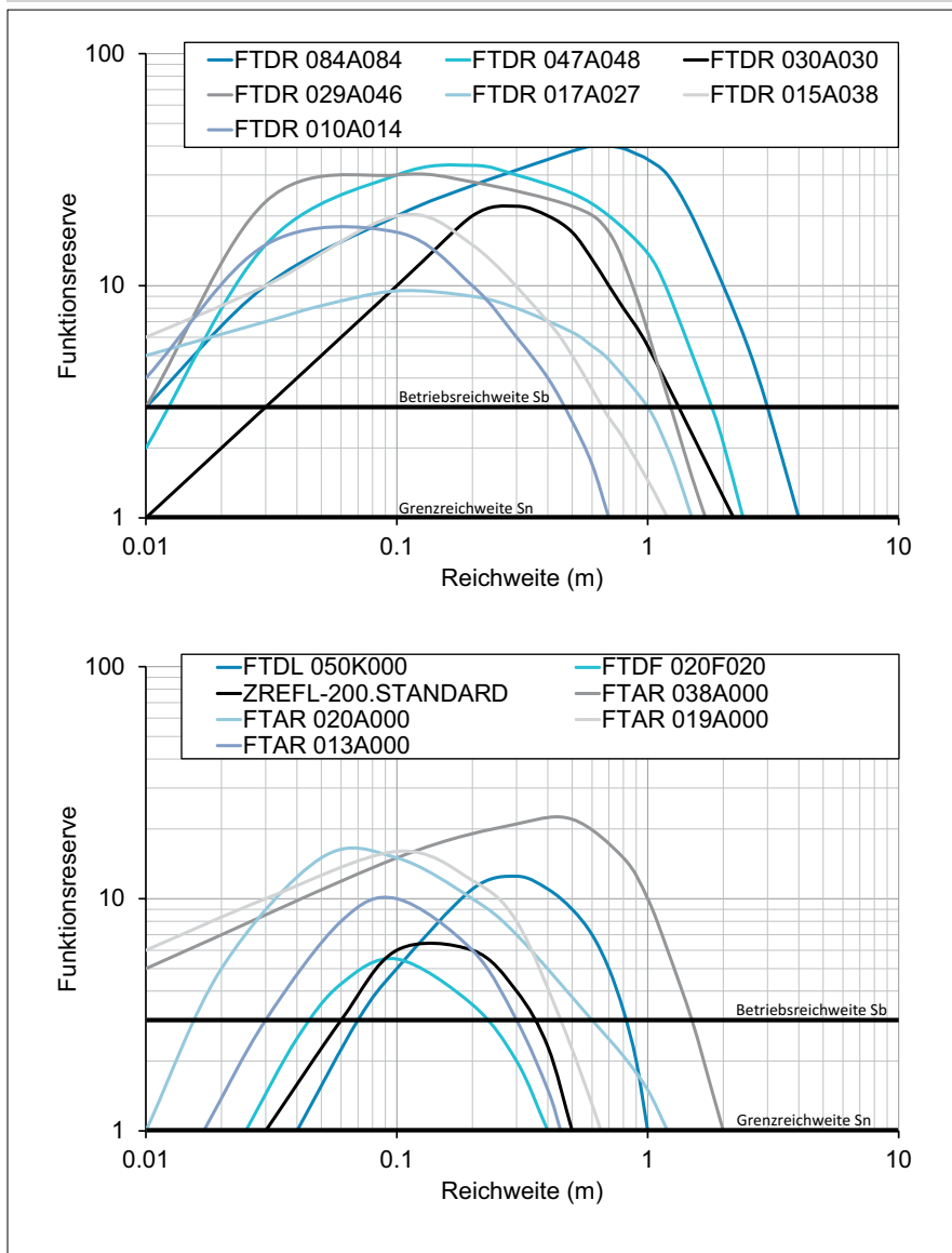
Funktionsreservekurven
