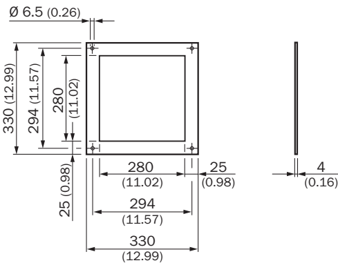
Rysunek wymiarowy (Wymiary w mm)
