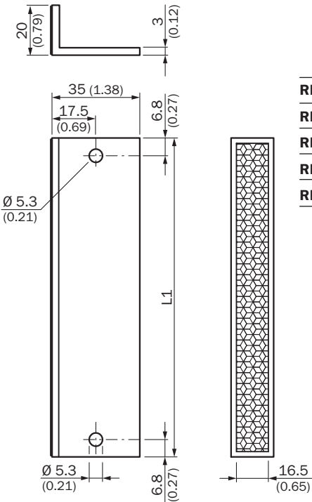
Rysunek wymiarowy (Wymiary w mm)
