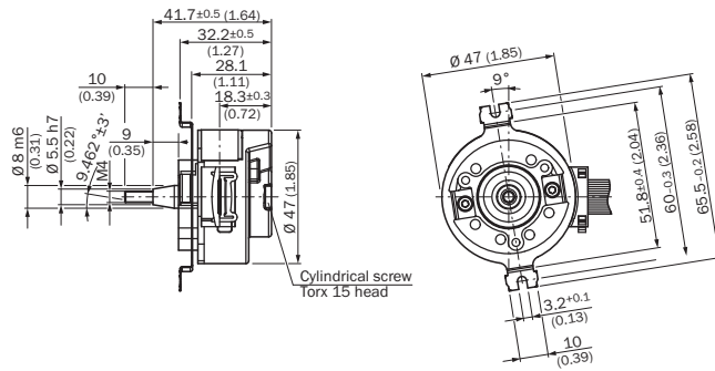
Rysunek wymiarowy (Wymiary w mm)
