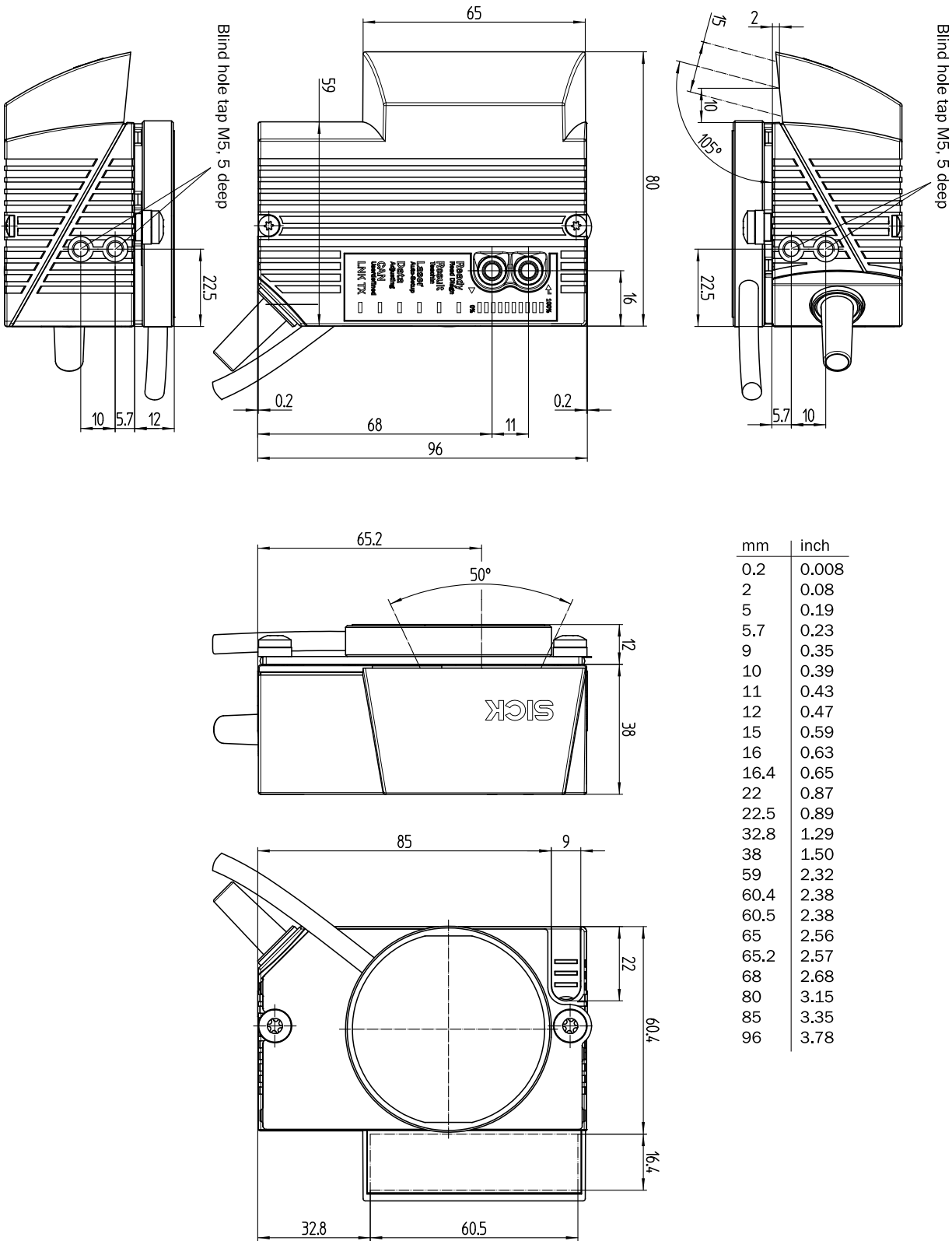
Rysunek wymiarowy (Wymiary w mm)
