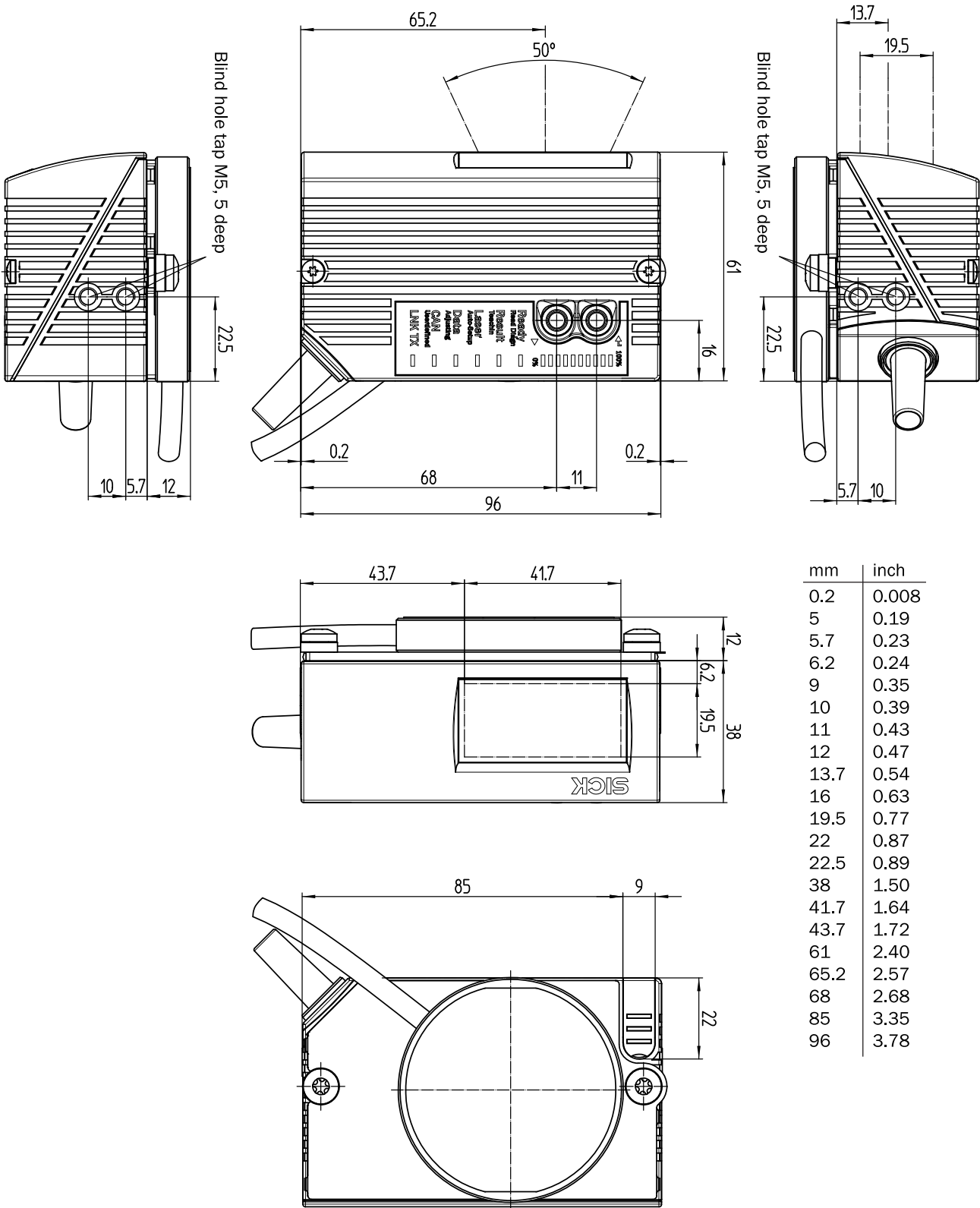
Rysunek wymiarowy (Wymiary w mm)
