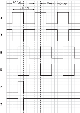
Сигнальные выходы для эл. интерфейсов TTL и HTL
