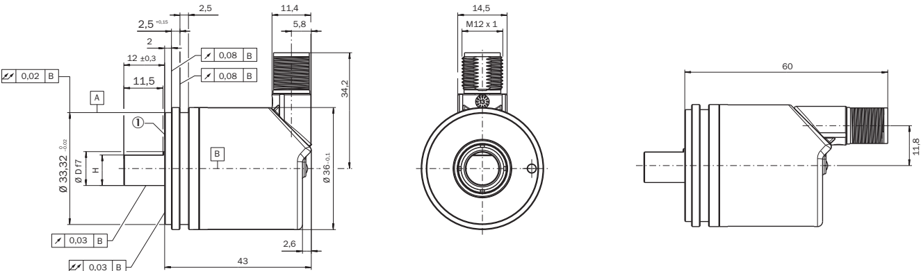
① Messpunkt für Betriebstemperatur
