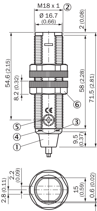
Габаритный чертёж (Размеры, мм) GRTE18, GRL18, GRSE18, пластмасса, кабель, осевой
