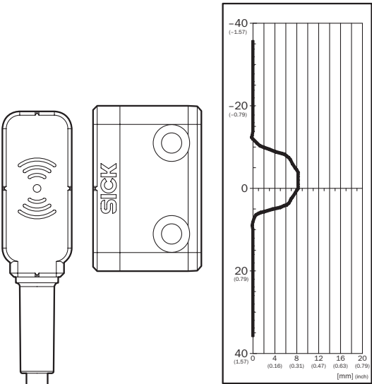
Безопасное расстояние включения S а0 6 мм
