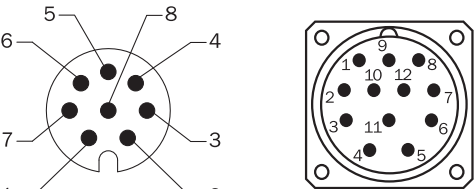
Ansicht Gerätestecker M12 / M23 an Leitung / Gehäuse
