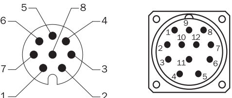
Widok wtyczki urządzenia M12/M23 na przewodzie/obudowie
