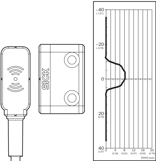
Безопасное расстояние включения S BO 6 мм
