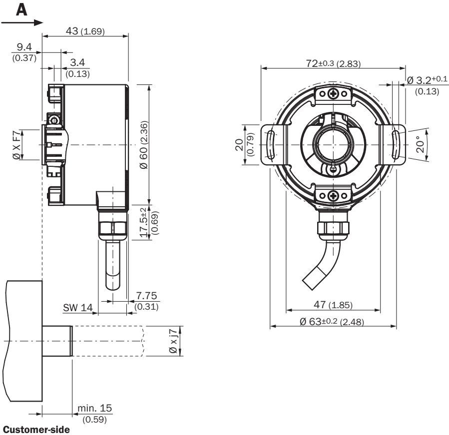
Габаритный чертеж (Размеры, мм)
