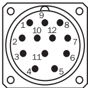
Ansicht Gerätesttecker M23 am Encoder
