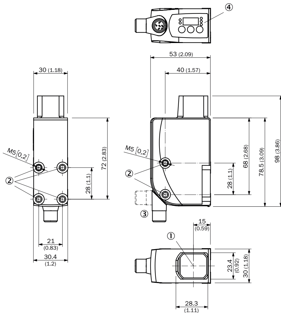
Rysunek wymiarowy (Wymiary w mm)
