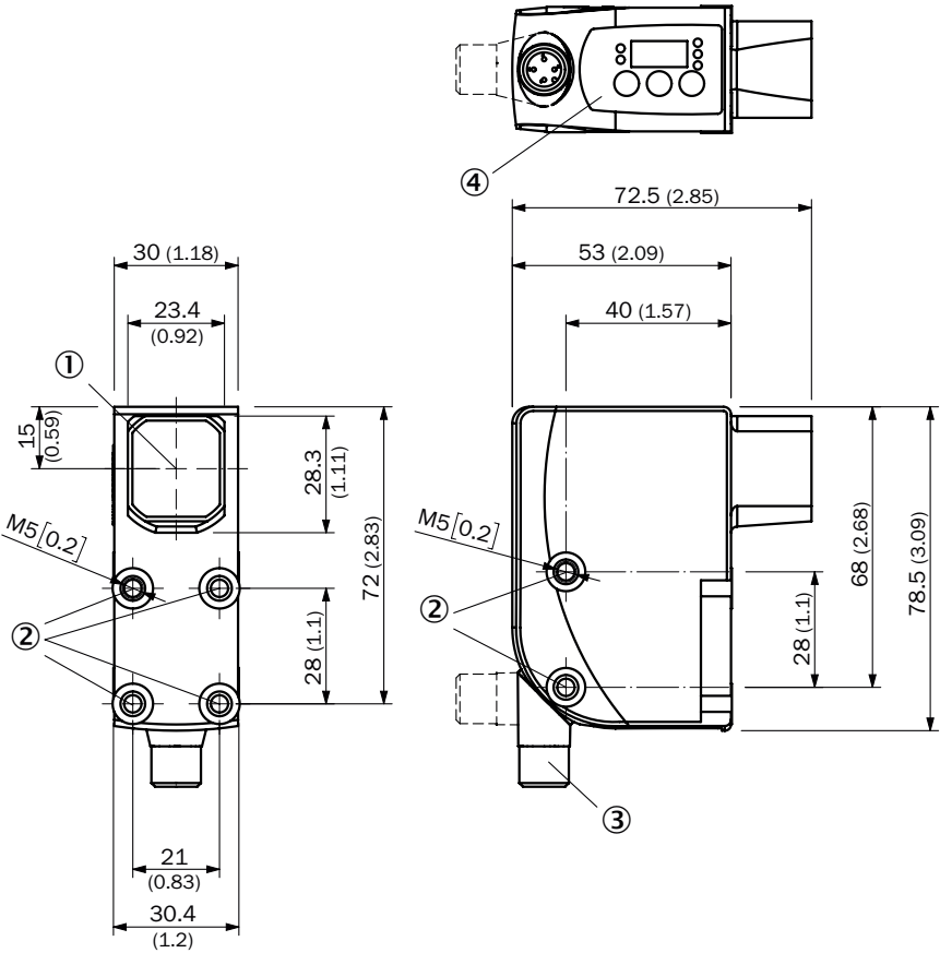
Габаритный чертёж (Размеры, мм)
