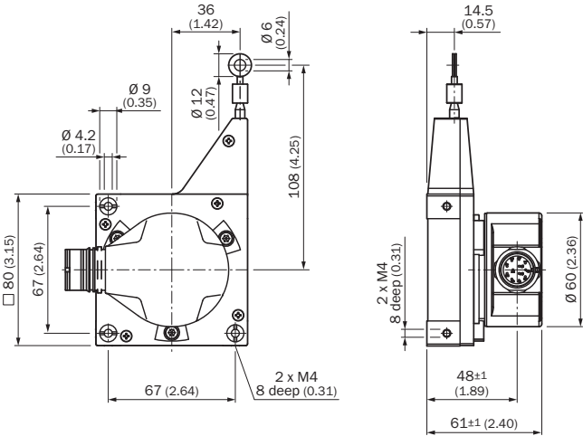
Rysunek wymiarowy (Wymiary w mm)
