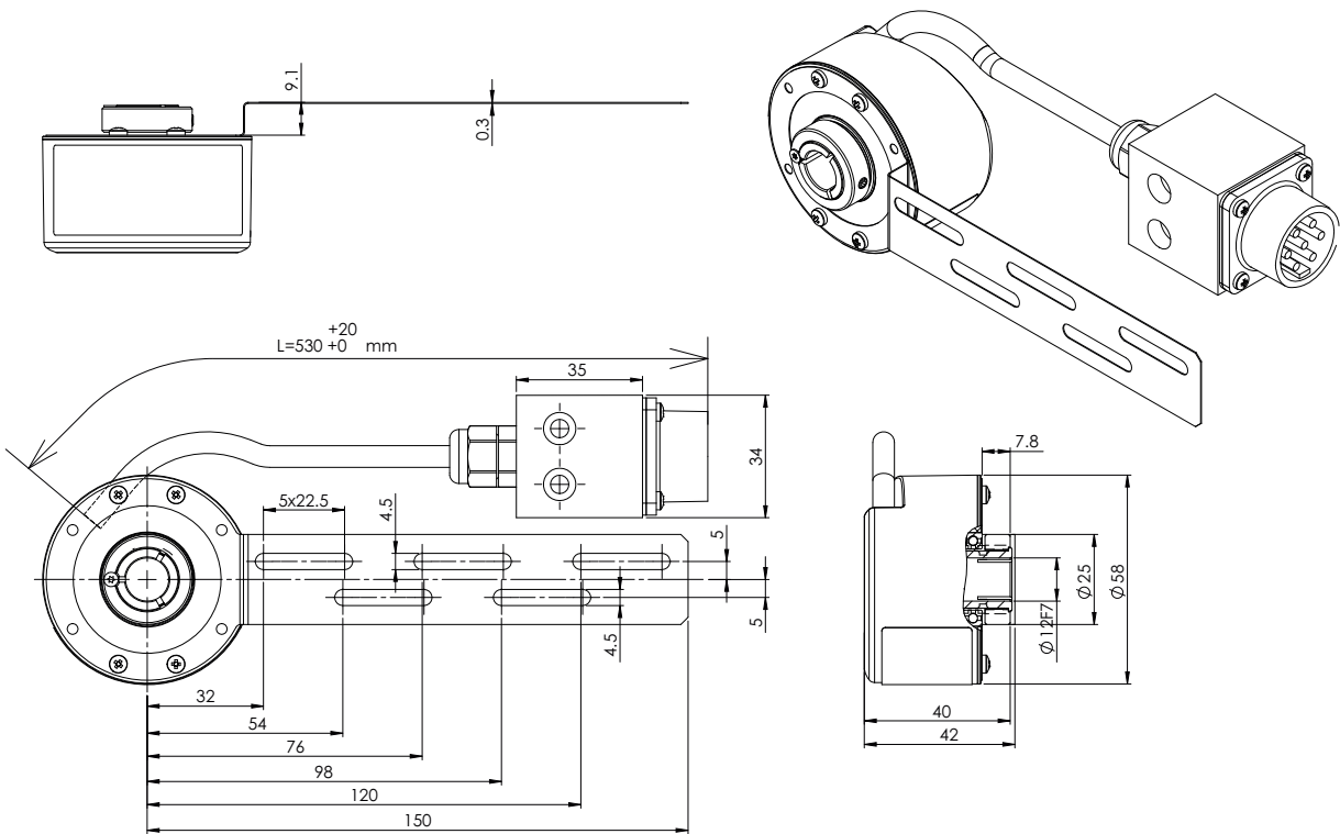
Rysunek wymiarowy (Wymiary w mm)
