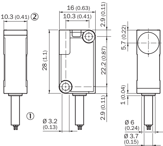
IQ10, cable
