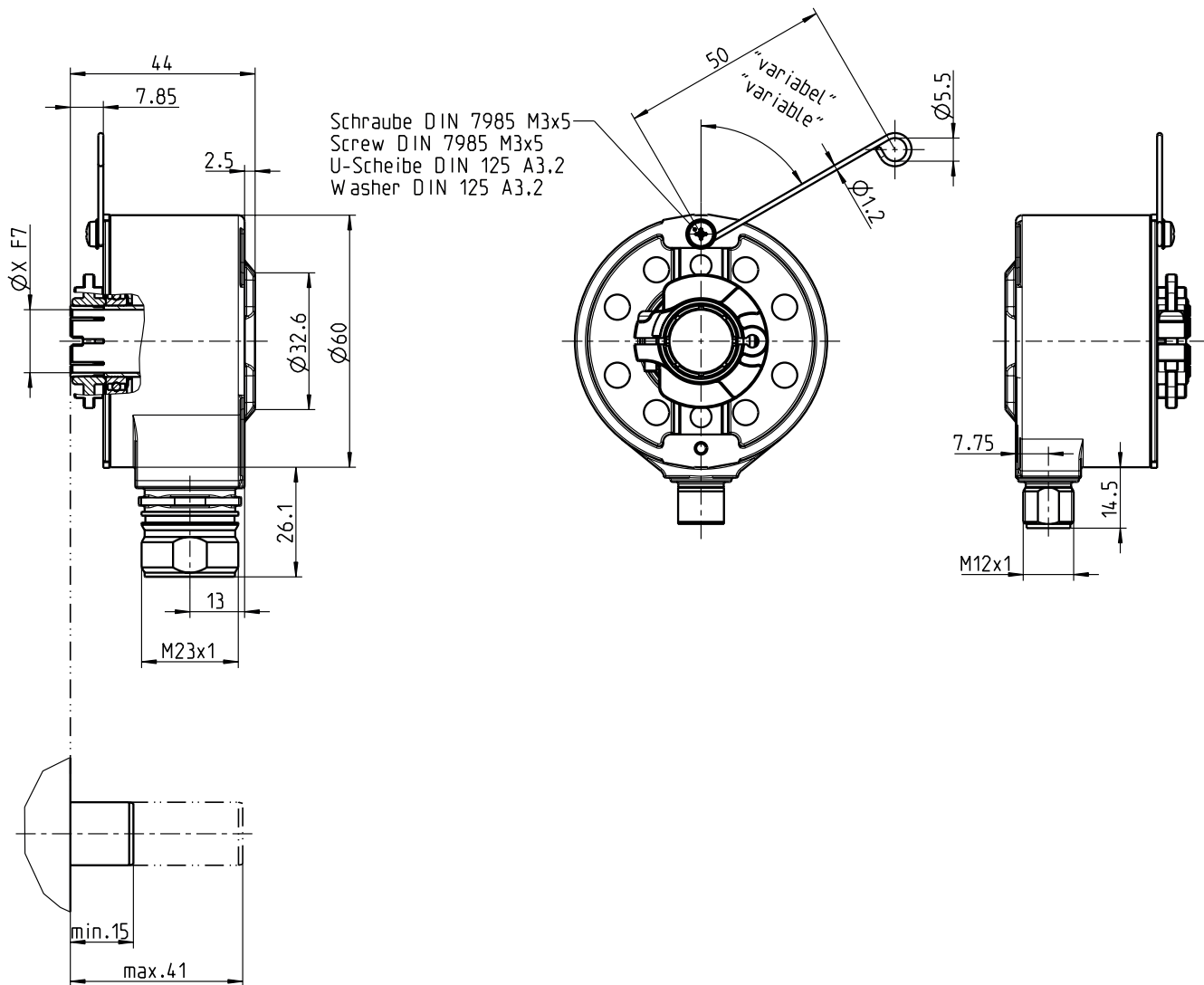
Rysunek wymiarowy (Wymiary w mm)
