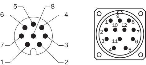
Widok wtyczki urządzenia M12/M23 na przewodzie/obudowie
