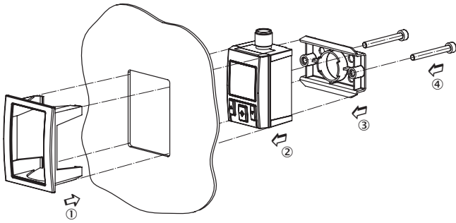
Zestaw mocujący
