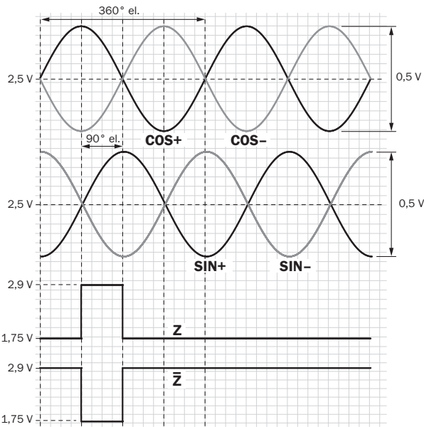
Bei Drehung der Welle im Uhrzeigersinn mit Blick in Richtung "A" (siehe Maßzeichnung)
