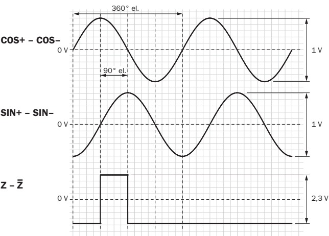
Bei Drehung der Welle im Uhrzeigersinn mit Blick in Richtung "A" (siehe Maßzeichnung) Schnittstellensignale SIN/COS vor Differenzbildung
