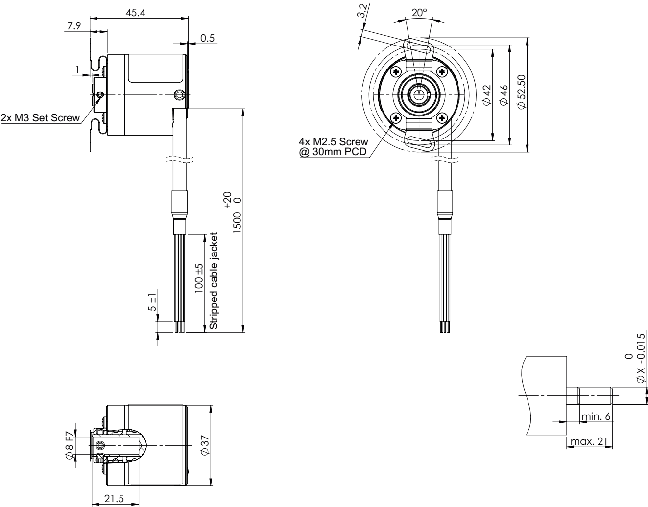
Rysunek wymiarowy (Wymiary w mm)
