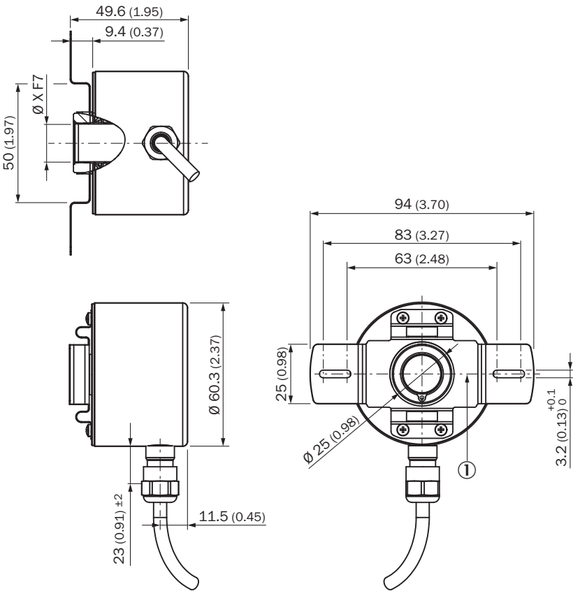
① Маркировка нулевого импульса на фланце
