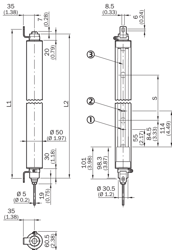
Rysunek wymiarowy (Wymiary w mm)
