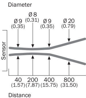
Размеры, мм
