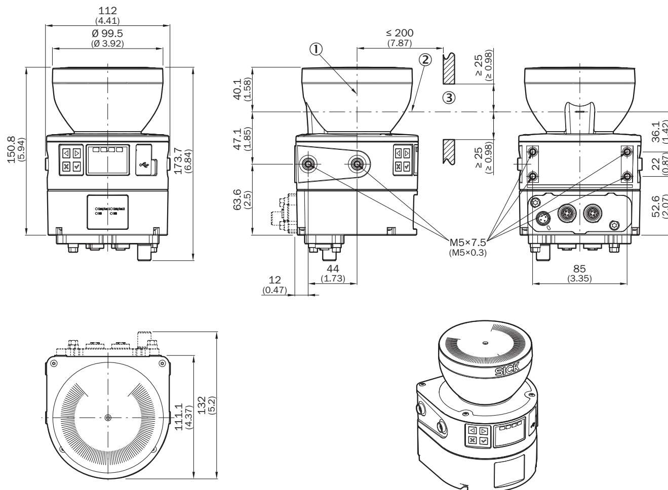
Rysunek wymiarowy (Wymiary w mm)
