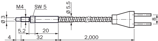
Габаритный чертеж (Размеры, мм)
