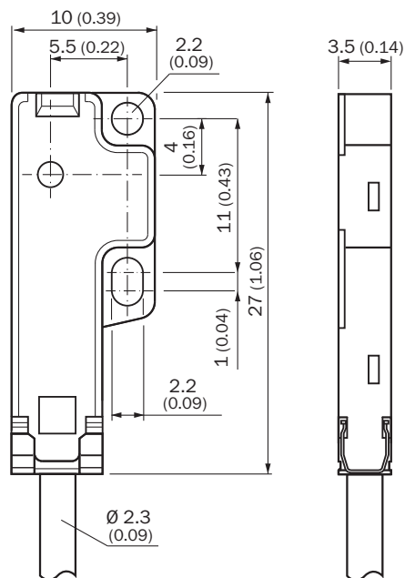
GSE2 Flat
