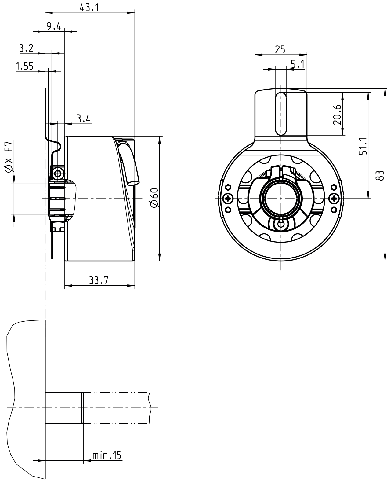
Rysunek wymiarowy (Wymiary w mm)
