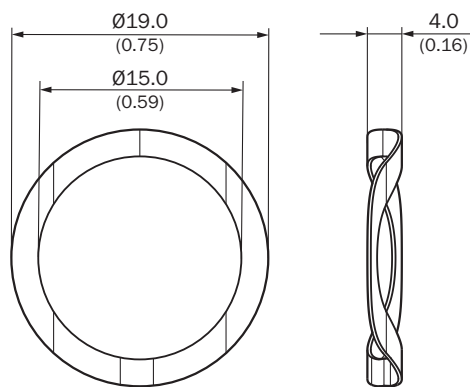
Волновая пружина
